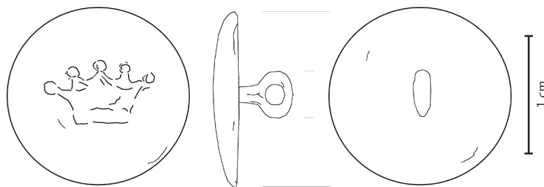
■ Obr. 4 Mosazný knoflík s reliéfem korunky s pěti perlami, hrob č. 1, jedinec č. 8, kresba M. Holas.
