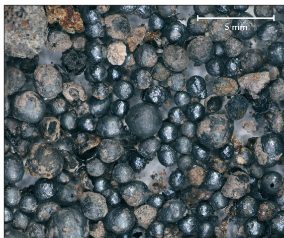
■ Obr. 6 Globulární okuje vzniklé při kovářském svařování.
