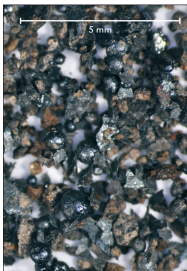
■ Obr. 7 Šupinky lamelárních okují vznikající na povrchu nahřívávaného předmětu.
