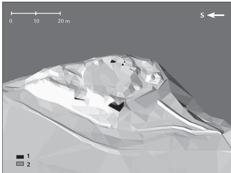
■ Obr. 8 Liběhrad, okr. Praha-západ. 3D model hradního jádra se šíjovým příkopem a dochovanými fragmenty zdiva v programu ATLAS. 1 zdivo, 2 zdivo v sekundární poloze.
