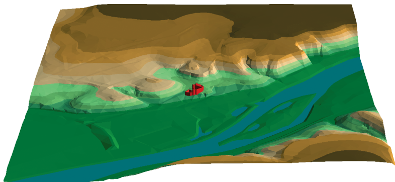
■ Obr. 4 3D modelace vltavského údolí a části okolního terénu s hradním areálem v programu ATLAS 9.
