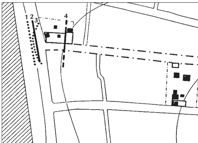
■ Obr. 4 Lübeck. Změny v topografickém vývoji v Přístavní a Obchodní čtvrti na Alfstrasse. 1 průběh nábřeží kolem r. 1217; 2 městská hradba kolem r. 1217; 3 průběh nábřeží kolem r. 1157; 4 průběh městské hradby kolem r. 1181 (Fehring 1994).
