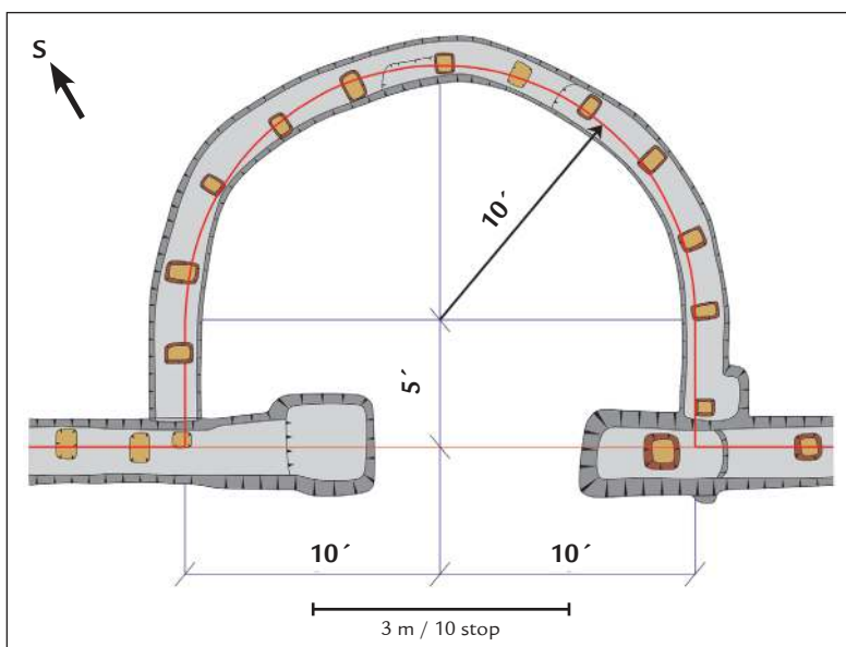
■ Obr. 6 Mušov-Neurissen, stavba s apsidou – detail základového žlábků vlastní apsidy. Vyznačena jsou lůžka v místech patek svislých trámů. Červené čáry reprodukuje rozměry půdorysné dispozice v intencích plánu připraveného římskými architekty. Rozměry jsou uváděny v římských stopách.
