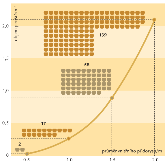
■ Obr. 9 Funkce vyjadřující vztah mezi průměrem vnitřního půdorysu pece a objemem peciště za předpokladu, že má peciště tvar polokoule. Graficky je znázorněna teoretická maximální vsádka nádob o výšce a maximální šířce vřutě 25 cm. Při průměru vnitřního půdorysu 0,5 m jsou to 2 nádoby, 17 nádob při průměru 1 m, 58 nádob při průměru 1,5 m a 139 nádob při průměru 2 m.
