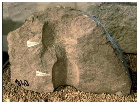
■ Obr. 3 Mlýnský kámen prasklý při vrtání středového otvoru. Patrné je vrtání dutým i špičatým vrtákem. Úprava na Kometě v Píseckých horách. Foto V. Komasová.
