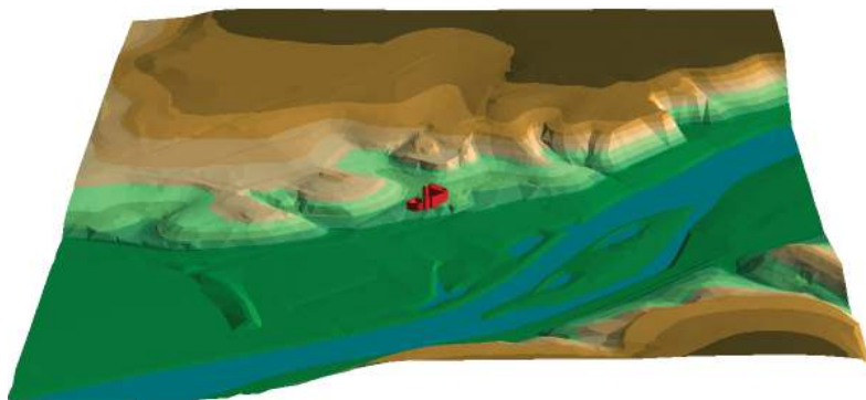
■ Obr. 4 3D modelace vltavského údolí a části okolního terénu s hradním areálem v programu ATLAS 9.
